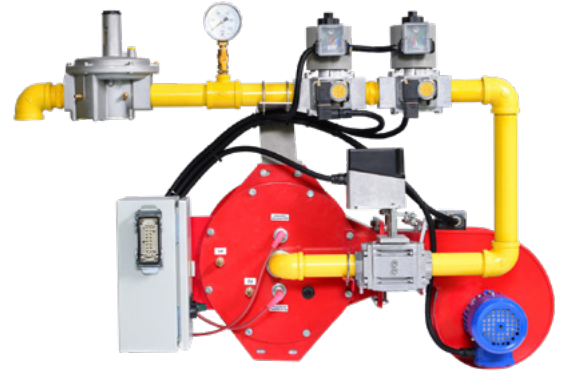
Yüksek Güçlü Brülör
