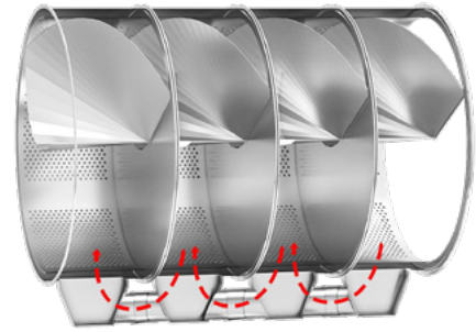
Su bir sonraki bölmeye alttan geriye doğru akar
