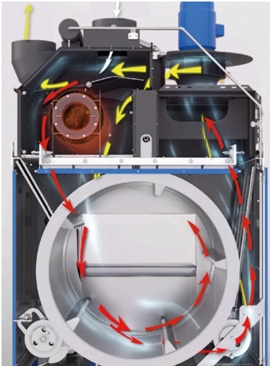
Geliştirilmiş Hava Sirkülasyon Sistemi
